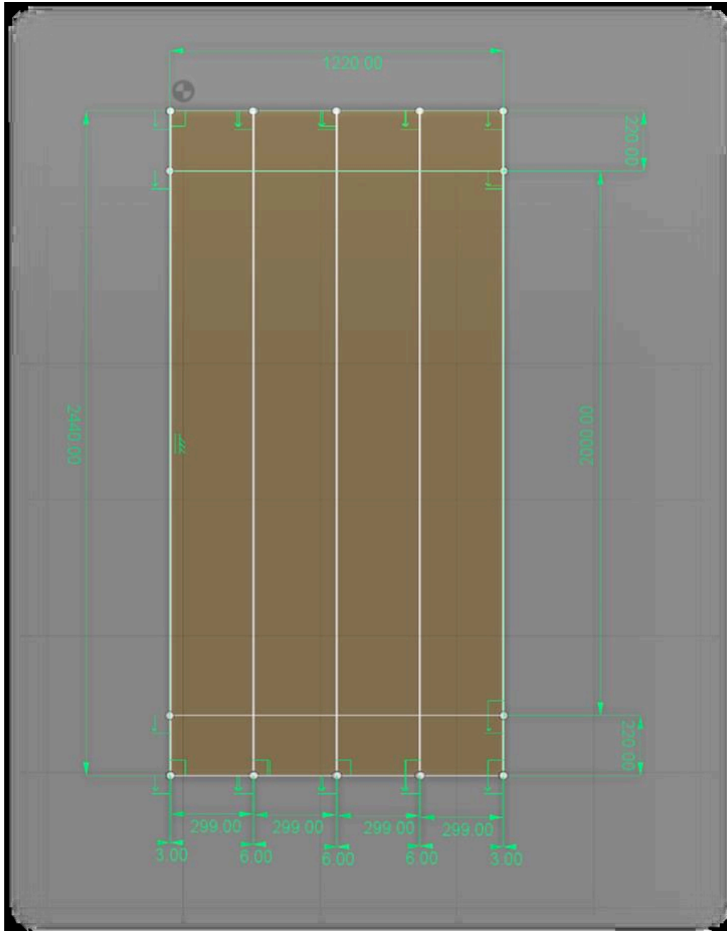
Medidas de la pista en milímetros
