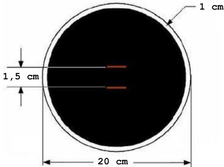
Figura 1. Medidas del Dohyo
